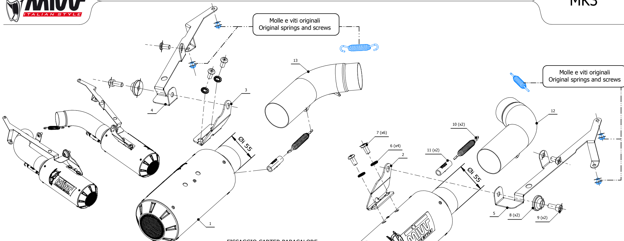
FISSAGGIO CARTER PARACALORE HEAT SHIELD FIXING
